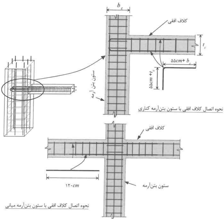
شکل ۷-۱۹: جزئیات میلگردگذاری برای اتصال کلاف افقی به ستون بتنی آرمه
