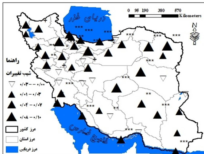
شکل ۶: شیب تغییرات آستانه‌های دمایی امواج سرمایی (***) معنی داری در سطح معنی‌داری ۰/۹۹۹، °° روند در سطح معنی‌داری ۹۹ درصد، ° روند در سطح معنی‌داری ۹۵ درصد، + روند در سطح معنی‌داری ۹۰ درصد، بدون علامت وجود روند در سطح معنی‌داری کمتر از ۹۰ درصد).
