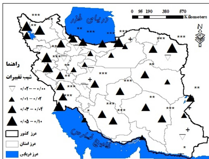
شکل ۷: شیب تغییرات آستانه‌های دمایی امواج گرمایی (***) معنی داری در سطح معنی‌داری ۰/۹۹۹، °° روند در سطح معنی‌داری ۹۹ درصد، ° روند در سطح معنی‌داری ۹۰ درصد، + روند در سطح معنی‌داری ۹۰ درصد، بدون علامت وجود روند در سطح معنی‌داری بیشتر از ۹۰ درصد).
