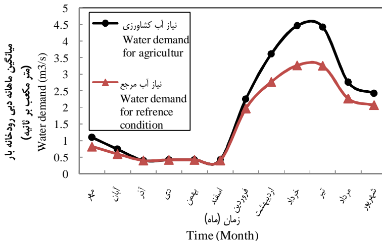
شکل 8- نیاز آبی ماهانه در سناریوهای افزایش سطح کشاورزی و مرجع تحت سناریوی A2
