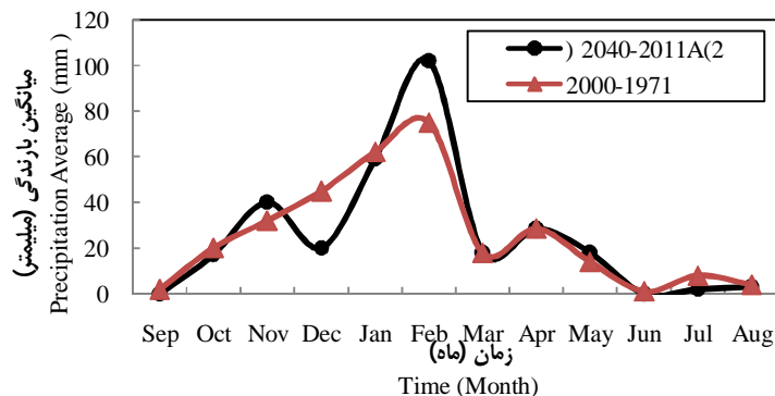
شکل 2- میانگین بارندگی ماهانه در دو دوره (1971-2000) و (2011-2040) در ایستگاه اریه Figure 2- Precipitation monthly average in periods of (1971- 2000) and (2011- 2040) in Arie station
