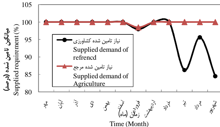
شکل 9- درصد نیاز تأمین شده در سناریوهای افزایش سطح کشاورزی و مرجع تحت سناریوی A2
