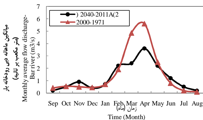
شکل 5- مقایسه میانگین ماهانه دبی رودخانه بار در دوره تنظیم و ارزیابی
