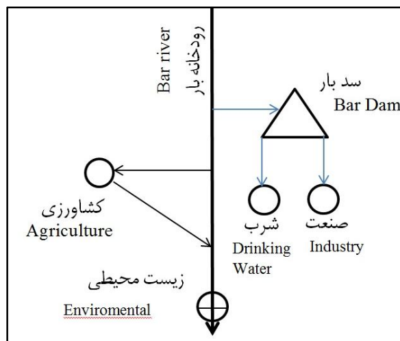
شکل 6- پیکربندی سیستم منابع آب رودخانه بار در مدل WEAP
