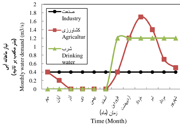
شکل 7- نیاز ماهانه آبی در سال پایه برای هر یک از نقاط نیاز در مدل WEAP
