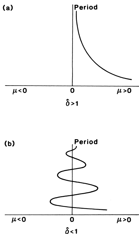
FIGURE 27.3.9. a) \delta > 1 . b) \delta < 1 .
