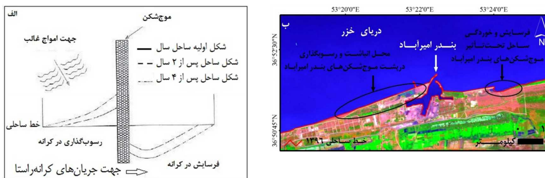
شکل ۹: الف) نمایی شماتیک از چگونگی تأثیر احداث و توسعه سازه‌های مهندسی (موج‌شکن) در تغییر وضعیت سواحل؛ ب) تأثیر احداث موج‌شکن و توسعه دستک‌های بندر امیرآباد در تغییر وضعیت کرانه‌های خاوری و باختری آن (LANDSAT, OLI Sensor, ۲۰۱۷).
