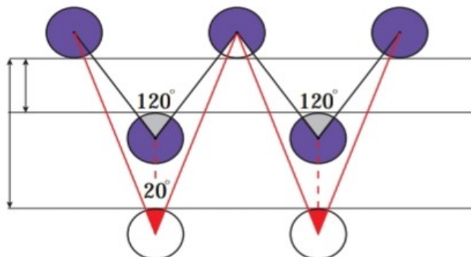
وضعیت قرار گیری تارها در شیوه نیم لول
