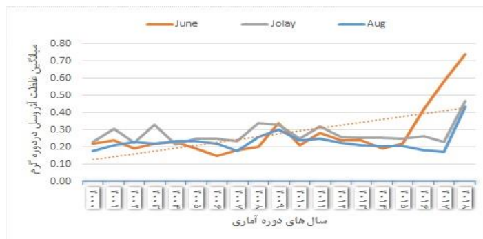
شکل ۷. نمودار میانگین روند تغییرات غلظت هواویزه در ماه ژوئن، جولای و اوت استان سیستان و بلوچستان (دوره آماری ۲۰۰۰ - ۲۰۱۸)
